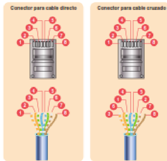
Fig. 2.20. Cable UTP normal y cruzado.
