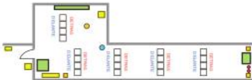
Fig. 2.26. Plano de instalación de armarios en un CPD.
