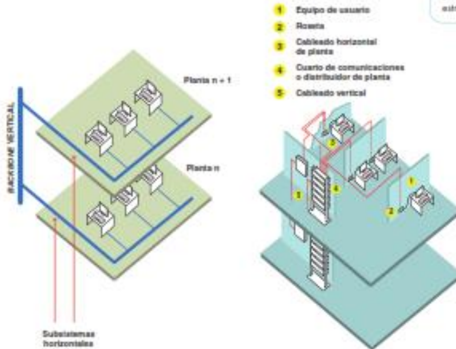
Fig. 3.33. Cableado estructurado vertical y horizontal en dos plantas de un edificio.
