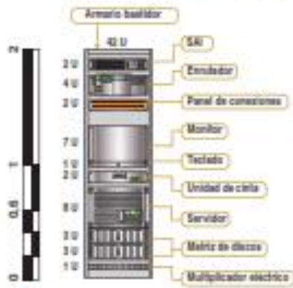
Fig. 2.15. Esquema de un armario. A la izquierda se ha representado una escala en metros.
