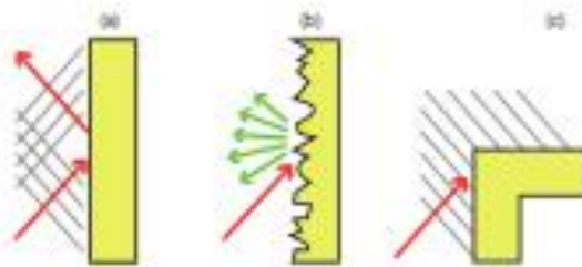
Fig. 1.3. Efectos de reflexión (a), dispersión (b) y difracción (c)
